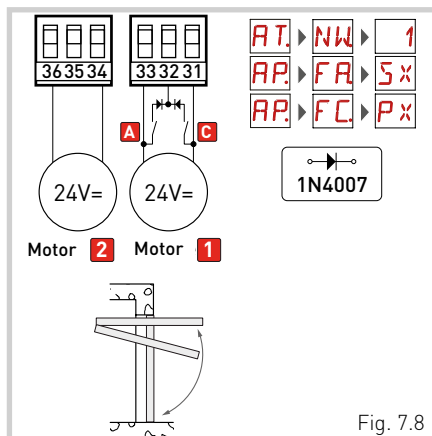
[Fig. 7.8] Installatie met elektrische eindschakelaars (stop tijdens sluiten en nadering tijdens sluiten)
